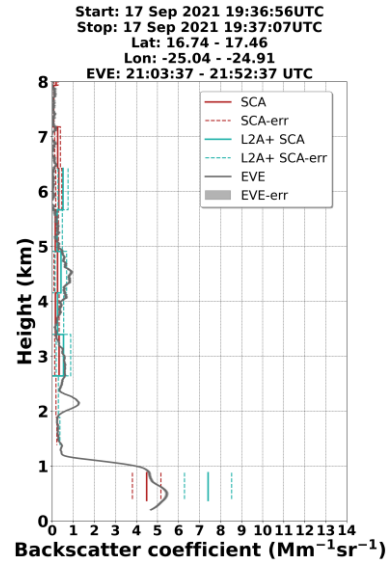
Aeolus b355nm – AEL-FM & MSG QA ( \text{Mm}^{-1}\text{sr}^{-1} )
