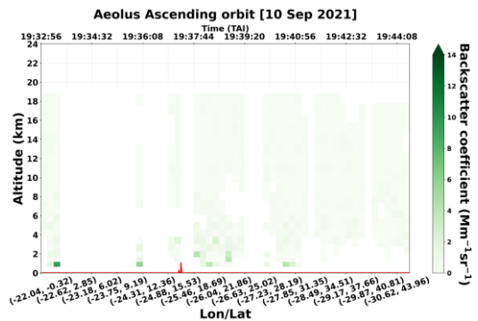
Aeolus b355nm – AEL-FM & MSG QA ( \text{Mm}^{-1}\text{sr}^{-1} )
