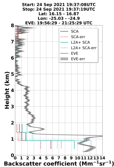
Aeolus b355nm – AEL-FM & MSG QA ( \text{Mm}^{-1}\text{sr}^{-1} )
