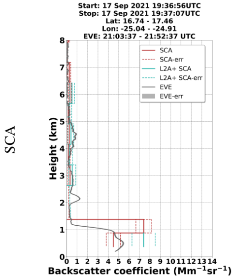
Aeolus b355nm ( \text{Mm}^{-1}\text{sr}^{-1} )
