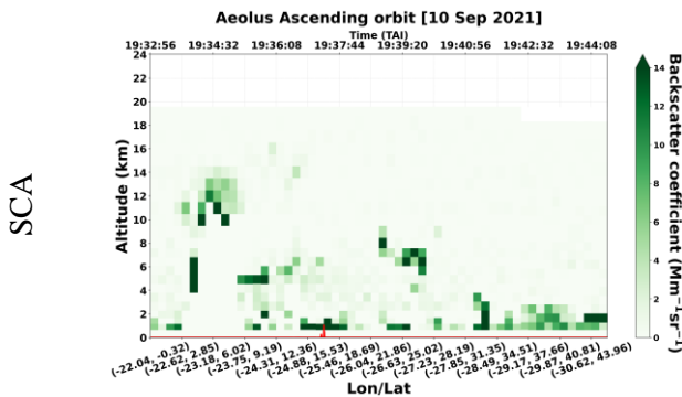
Aeolus b355nm - Raw ( \text{Mm}^{-1}\text{sr}^{-1} )
